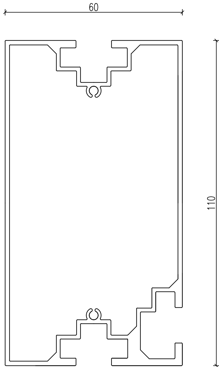
Profil 100.005
